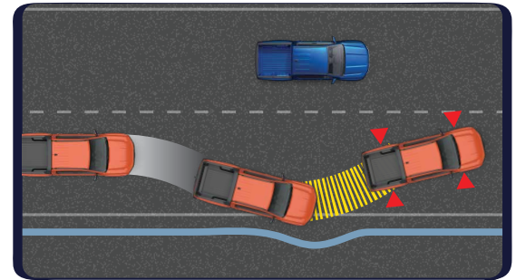
ប្រព័ន្ធចាប់ប្រឆាំងបន្ទាន់ដោយស្វ័យប្រវត្ត ក្រោយពេលមានការប៉ះទង្គិច
